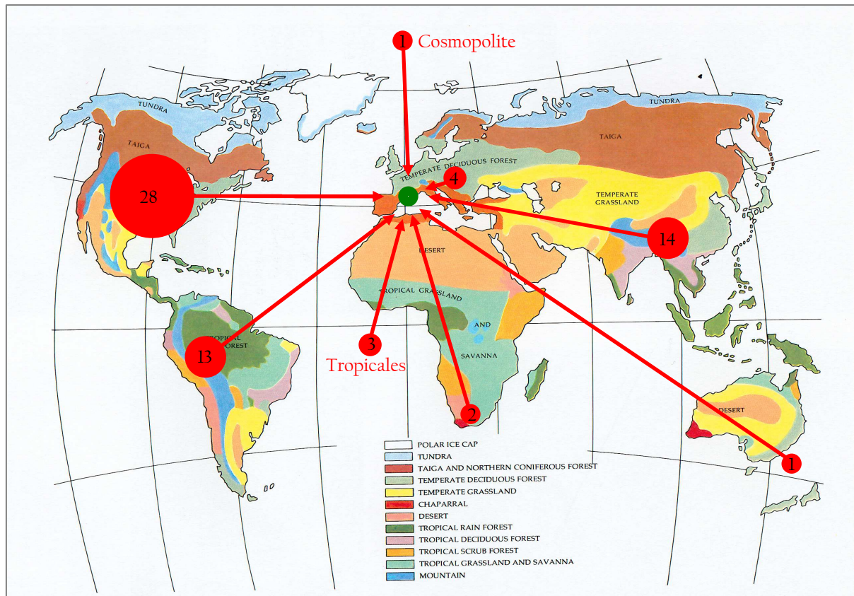
Figure 8 : Répartition des espèces en fonction de leur origine géographique
